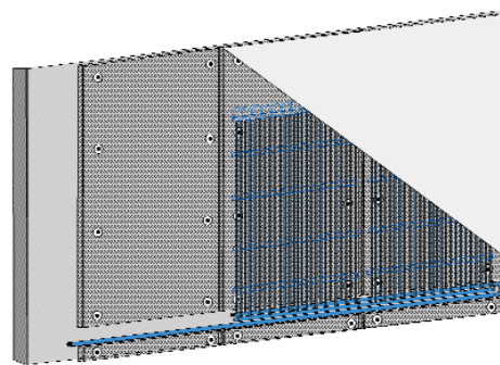
Fig. 1: Disposición de los colectores y tuberías según "Tichelmann" mediante el uso de placas de aislamiento para la formación de ranuras de instalación.
